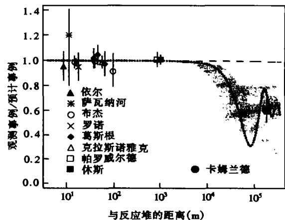
图 2 反应堆实验所得中微子通量的观测值与预期值之比。虚线代表太阳中微子没有振荡, 点线代表太阳中微子振荡“大角度混合解”, 阴影表示在 95% 的置信度下大角度混合解的允许范围
